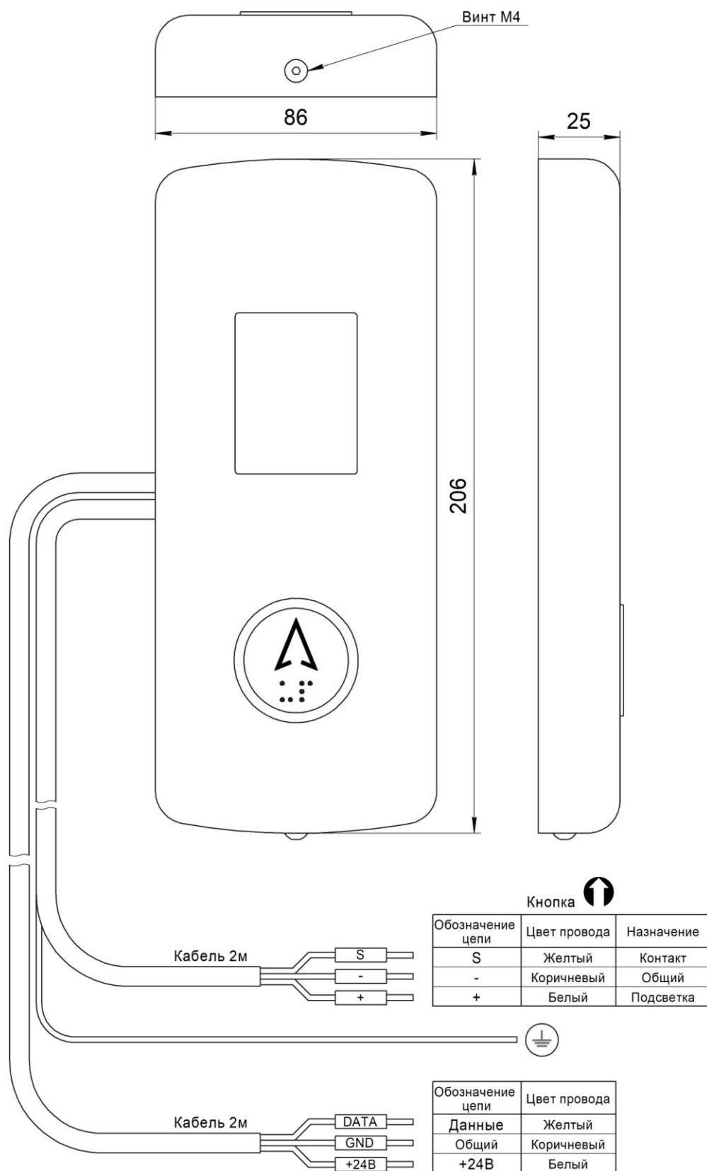
Рис.1 Внешний вид, габаритные и установочные размеры Вызывного поста ВП-1101-1074-07
